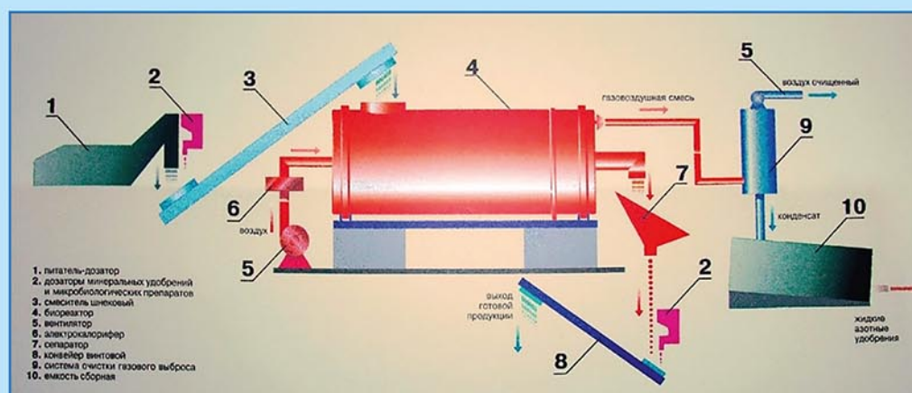
Технологическая схема переработки органического сырья во вращающихся барабанах.
